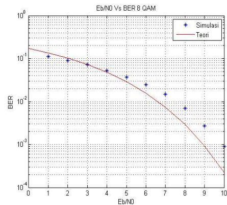
Gambar 12. Grafik Perbandingan E_b/N_0 terhadap BER 8-QAM
