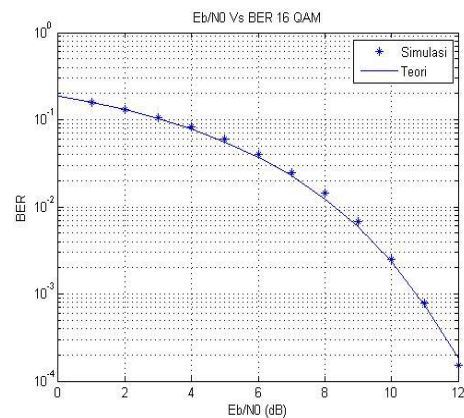
Gambar 13. Grafik Perbandingan E_b/N_0 terhadap BER 16-QAM
