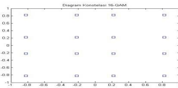
Gambar 10. Bentuk Konstelasi Diagram 16-QAM
