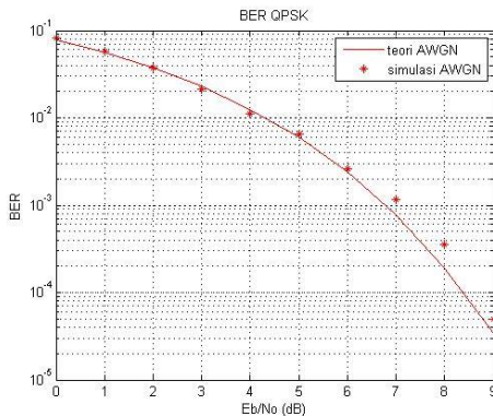
Gambar 11. Grafik Perbandingan E_b/N_0 terhadap BER QPSK
