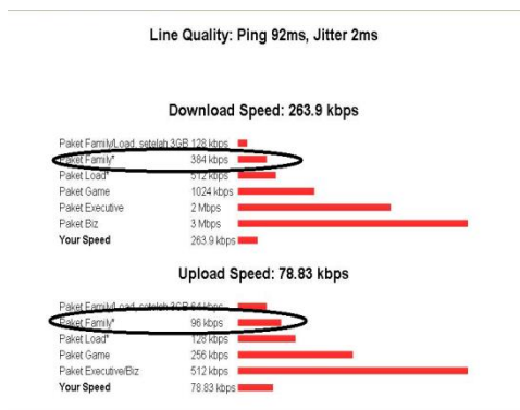
Gambar 12. Data speedtest
