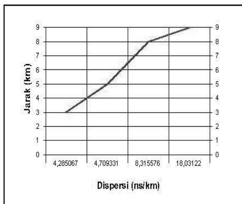
Gambar 8. Grafik Hubungan Antara Dispersi dengan Fibertype Singlemode
