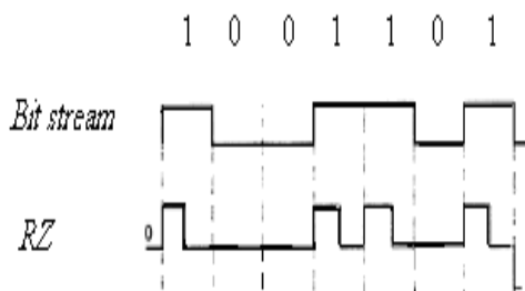
Gambar 3. Format kode RZ
