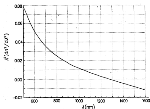
Gambar 1. Grafik \left| \lambda^2 d^2 n_1 / d\lambda^2 \right| vs. panjang gelombang
