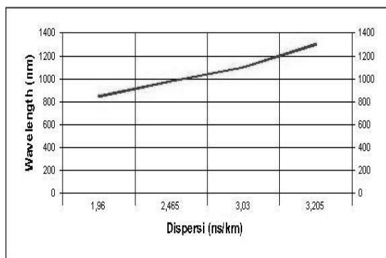
Gambar 6. Grafik Hubungan Antara Dispersi dengan Wavelength
