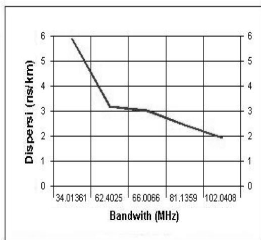
Gambar 12. Grafik Hubungan Antara Dispersi pada Fibertype Singlemode dengan Bandwidth
