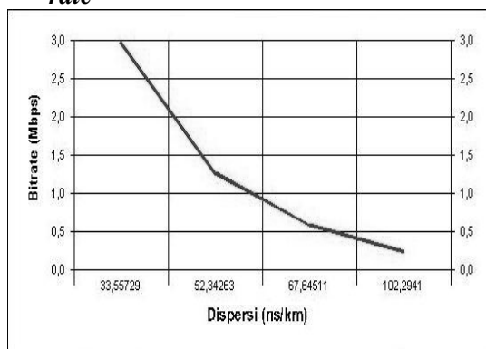
Gambar 4. Grafik Hubungan Antara Dispersi dengan Bit rate
