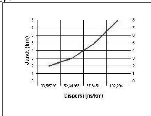
Gambar 7. Grafik Hubungan Antara Dispersi dengan Fibertype Multimode
