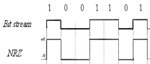
Gambar 2. Format kode NRZ
