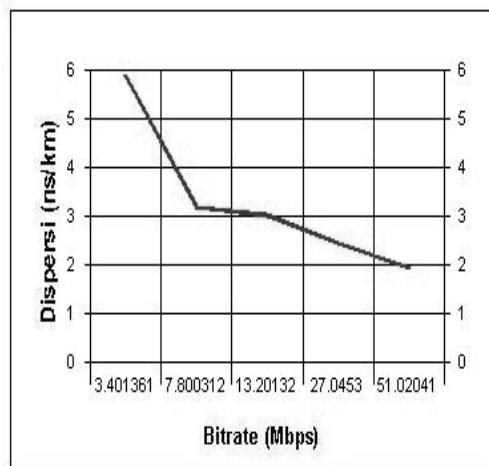
Gambar 10. Grafik Hubungan Antara Dispersi pada Fibertype Singlemode dengan Bit rate
