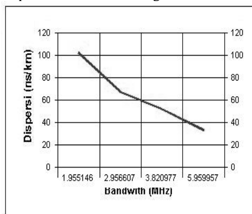
Gambar 11. Grafik Hubungan Antara Dispersi pada Fibertype Multimode dengan Bandwidth
