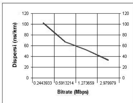
Gambar 9. Grafik Hubungan Antara Dispersi pada Fibertype Multimode dengan Bit rate
