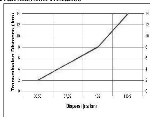
Gambar 5. Grafik Hubungan Antara Dispersi & Transmission Distance
