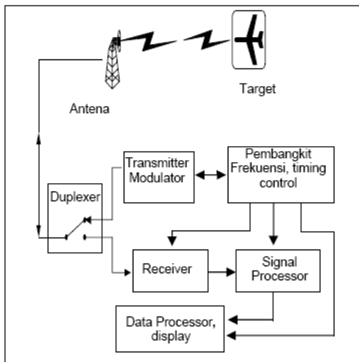
Gambar 4. Blok Diagram Prinsip Kerja Radar
