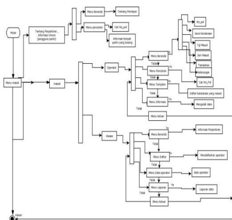
Gambar 12. Struktur Program
