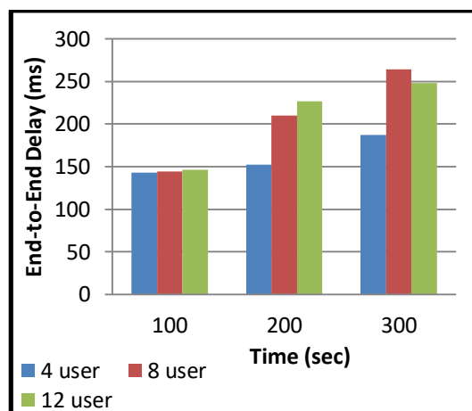
Gambar 20. Grafik End-to-End Delay pada Skenario Intserv
