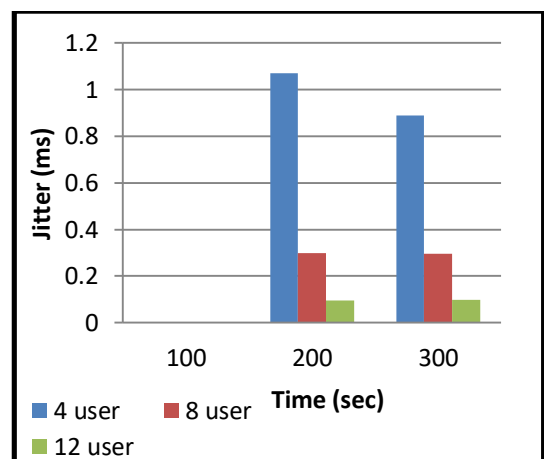
Gambar 25. Grafik Jitter pada Skenario Diffserv
