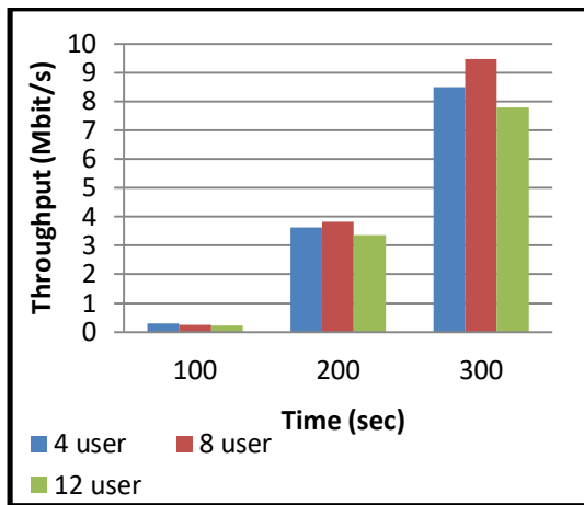
Gambar 23. Grafik Throughput pada Skenario Diffserv
