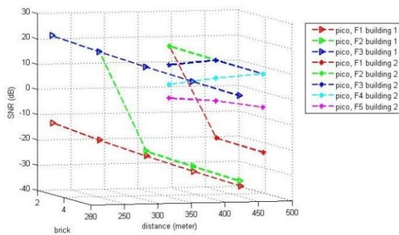
Fig. 7. SNR Picocell
