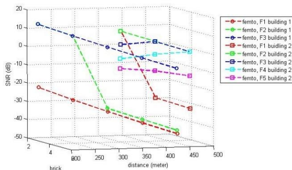
Fig. 5. SNR Femtocell
