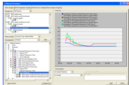
Gambar 17 Response Download dan Upload FTP Guerin dan Lucent (Poisson dengan Qos Beda)
