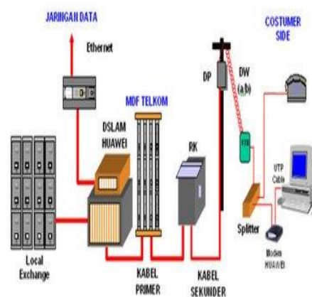
Gambar 1 Konfigurasi Jaringan ADSL
