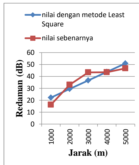
Gambar 5 Grafik jarak terhadap redaman nilai dengan metode Least Square vs nilai sebenarnya
