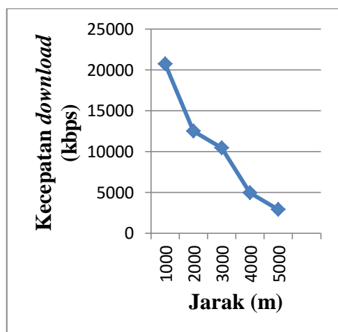
Gambar 4 Grafik jarak terhadap kecepatan download
