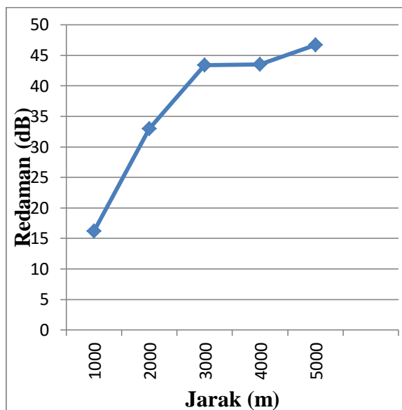
Gambar 2 Grafik jarak terhadap redaman
