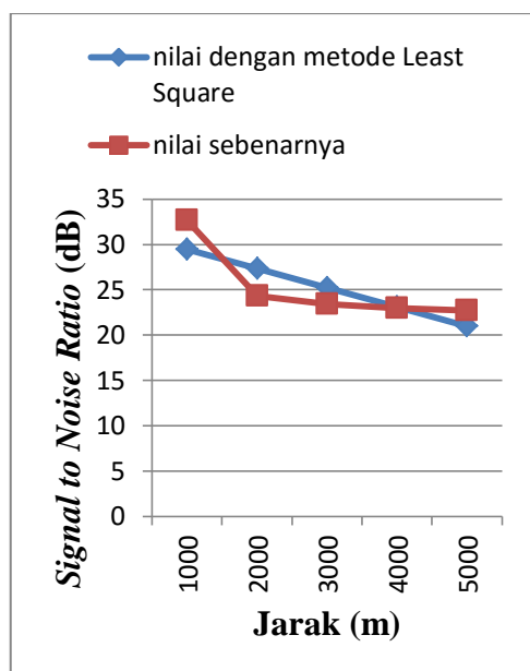
Gambar 6 Grafik jarak terhadap SNR nilai dengan metode Least Square vs nilai sebenarnya
