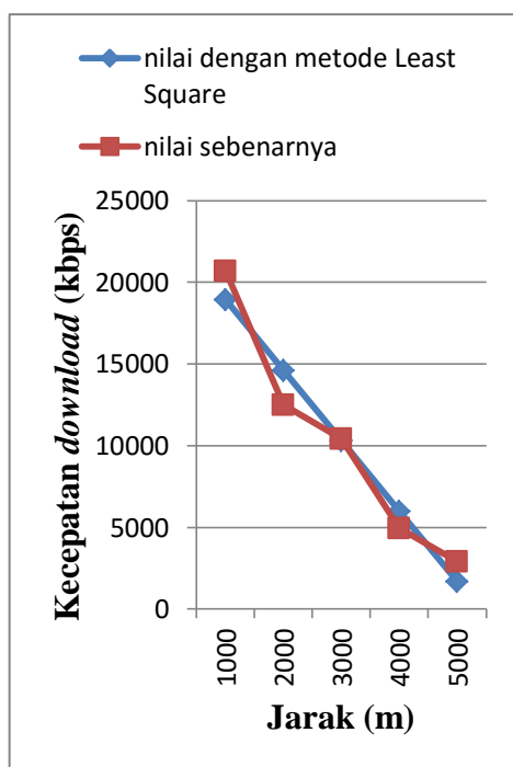
Gambar 7 Grafik jarak terhadap kecepatan download nilai dengan metode Least Square vs nilai sebenarnya
